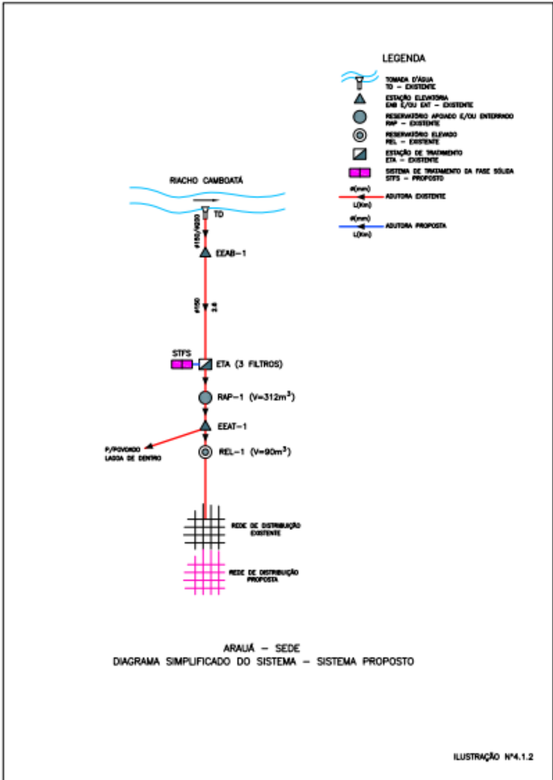
Figura 7 - Sistema Proposto
