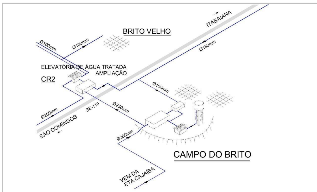
Figura 6 - Sistema de abastecimento de Campo do Brito
