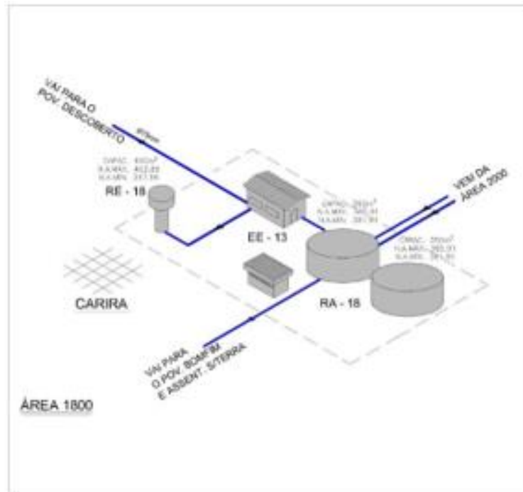
Figura 8 - Configuração do sistema de Carira
