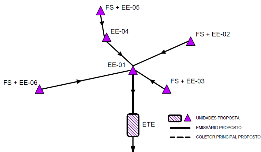
Figura 8 - Sistema de interligação das elevatórias
