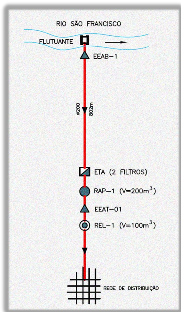
Figura 6 - Diagrama simplificado do sistema Ilha das Flores – SEDE
