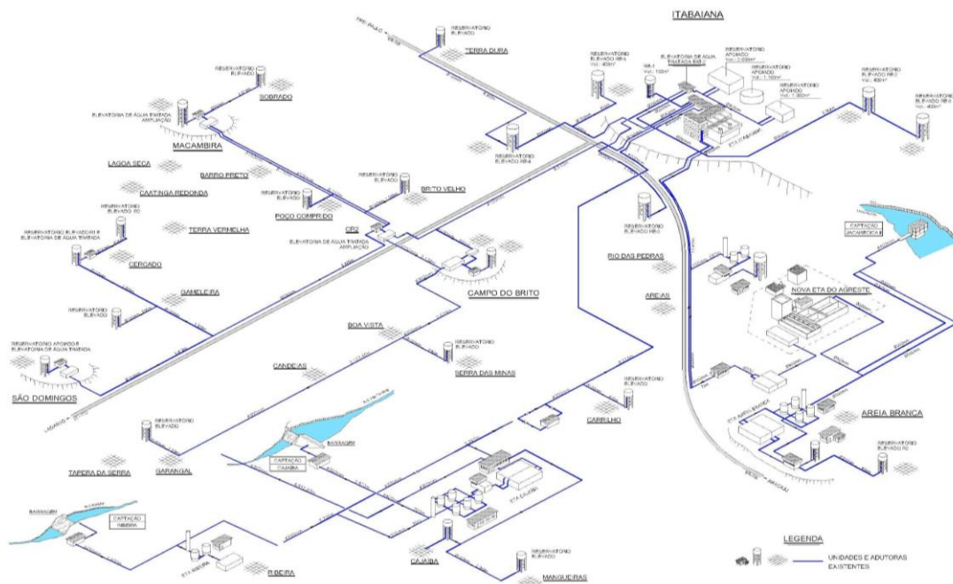
Figura 6 - Sistema Integrado da Adutora do Agreste
