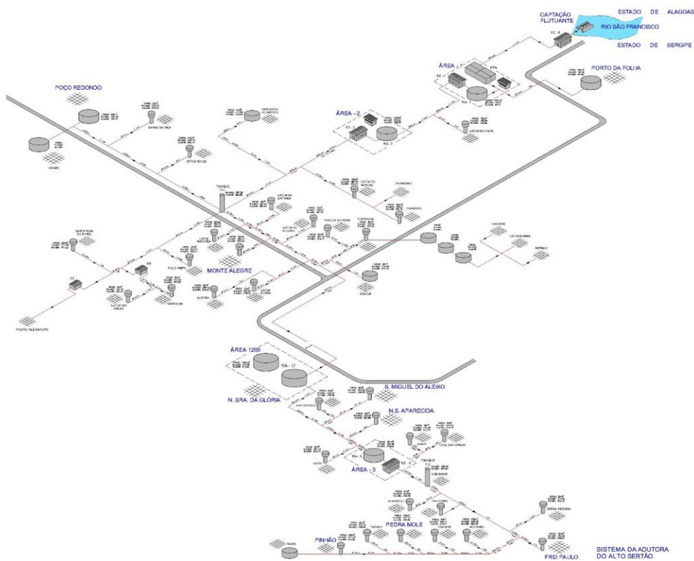
Figura 7 - Sistema Integrado da Adutora do Alto Sertão
