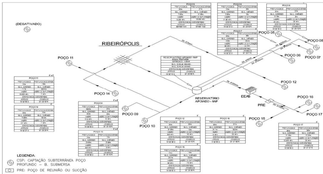
Figura 6 - Sistema de Abastecimento do município de Ribeirópolis
