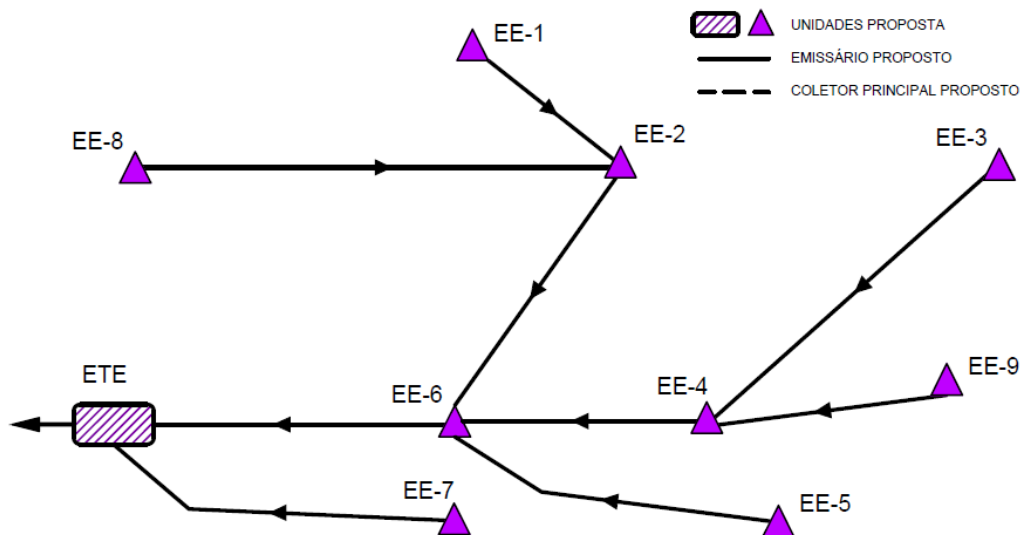
Figura 8 - Sistema de interligação das elevatórias
