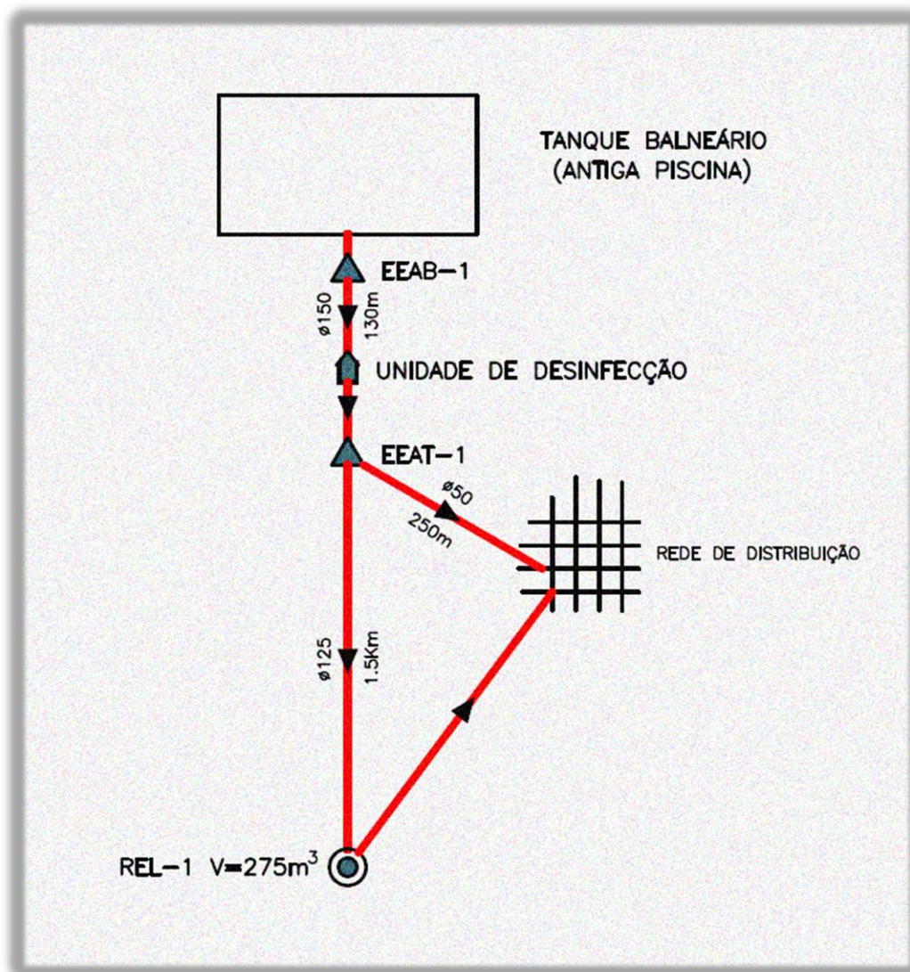
Figura 6 - Diagrama simplificado do sistema Salgado – SEDE
