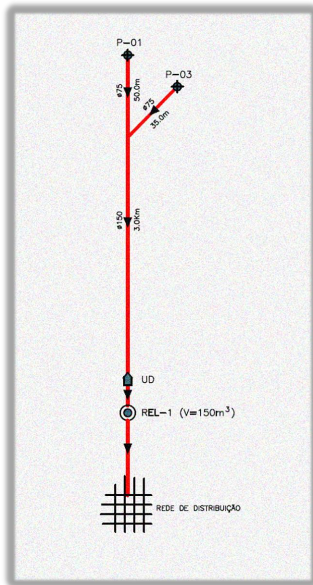
Figura 6 - Diagrama simplificado do sistema Santa Luzia do Itanhú – SEDE
