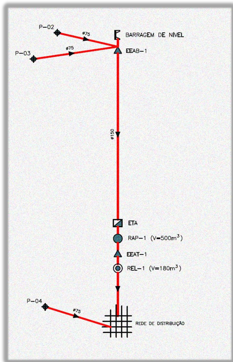
Figura 6 - Diagrama simplificado do sistema Santo Amaro das Brotas – SEDE
