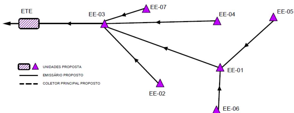
Figura 8 - Sistema de interligação das elevatórias
