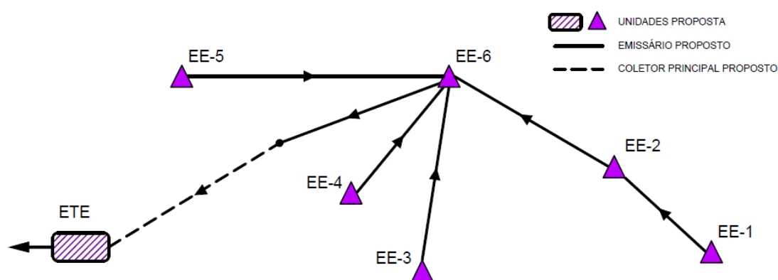
Figura 6 - Sistema de interligação das elevatórias
