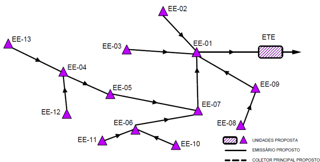
Figura 6 - Sistema de interligação das elevatórias
